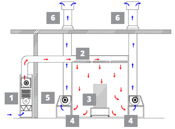
Gösterilen Model: YK-SO Kapalı Oda Kuru filtreli Yaş Boya Kabini Shown model: YK-SO Enclosed Dry Filtered Spray Paint Booth
