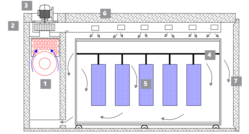
Shown model: TBF 400 Natural gas heated box type oven Gösterilen Model: TBF 400 Doğalgaz ısıtmalı kutu tipi fırın
